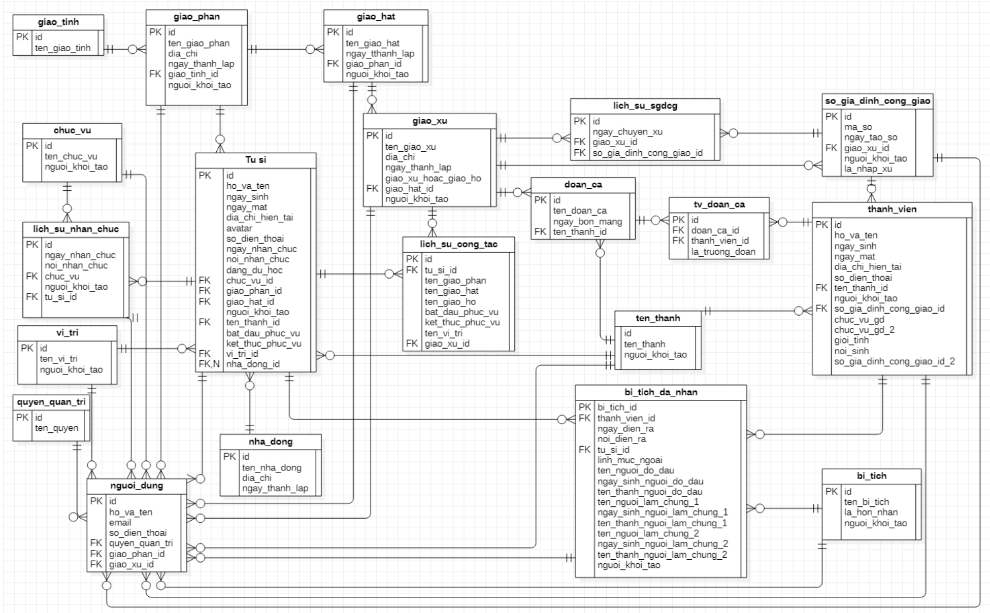
Hình 2.16 Mô hình ERD.
