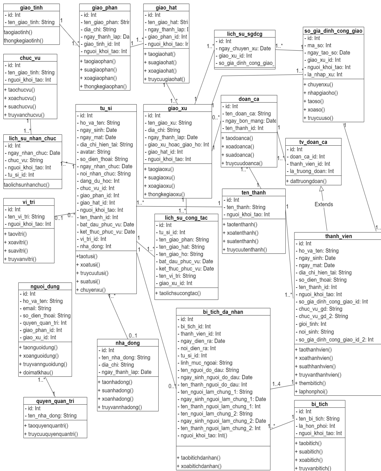
Hình 2.15 Mô hình lớp.
